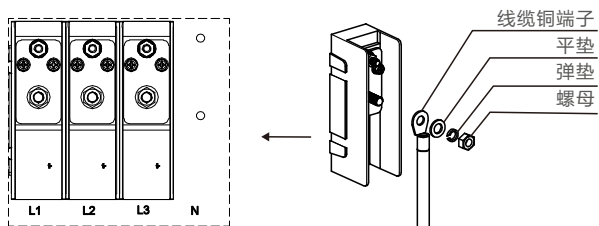
图3.20 铜铝过渡转接端子
