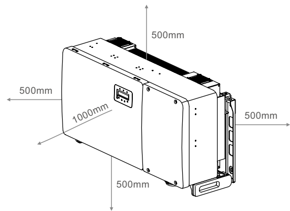
图3.1 逆变器的安装间隙
