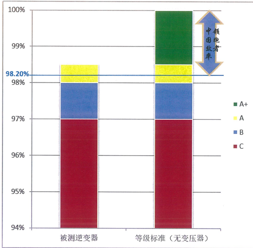
图 1. 逆变器效率水平对比图示
